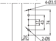
Middle pivot hinge
