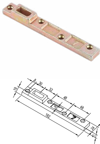
BJDP1103 中心摇臂 Center Pivoted Arm
