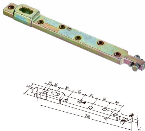
BJDP1303 中心摇臂 Center Pivoted Arm
