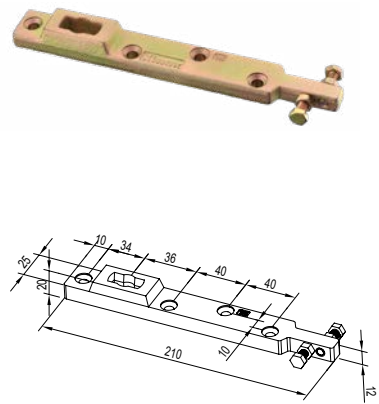
ZY01 中心摇臂 Center Pivoted Arm
