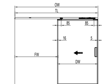
T1L14 移门拉手 Door handle
